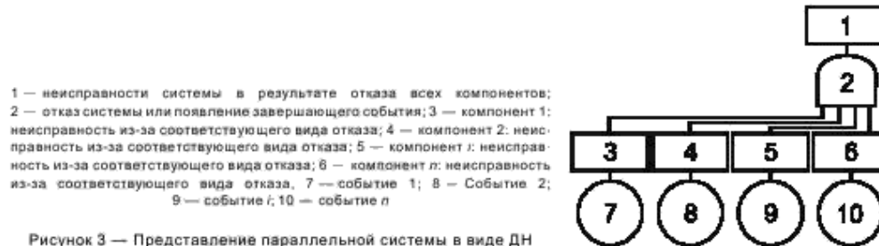
Рисунок 3 — Представление параллельной системы в виде ДН
