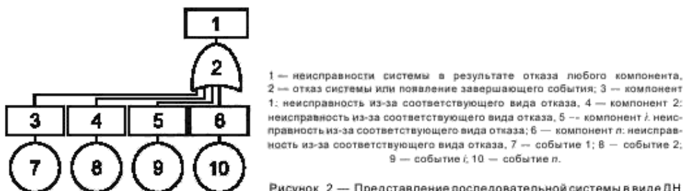
Рисунок 2 — Представление последовательной системы в виде ДН
