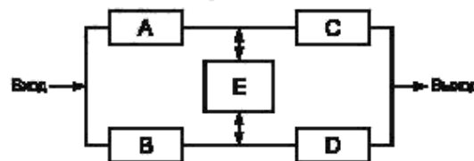
Рисунок 8 — Пример мостовой схемы, анализируемой с помощью ДН
