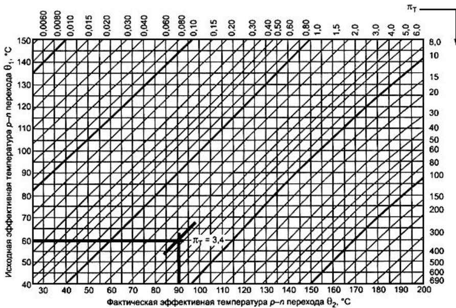
Рисунок А.1 - Зависимость интенсивности отказов от температуры
