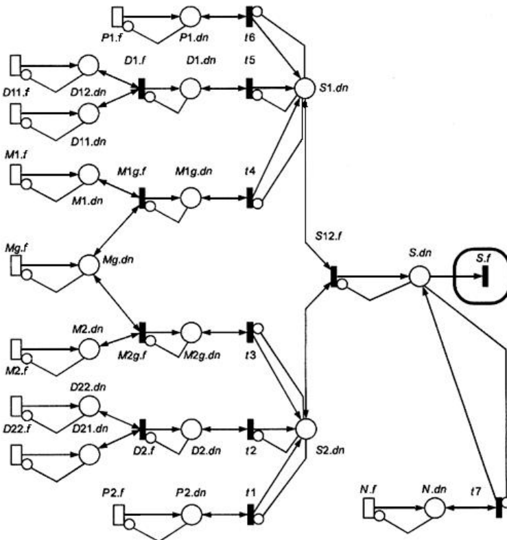
Рисунок А.9 - Сеть Петри мультипроцессорной системы
