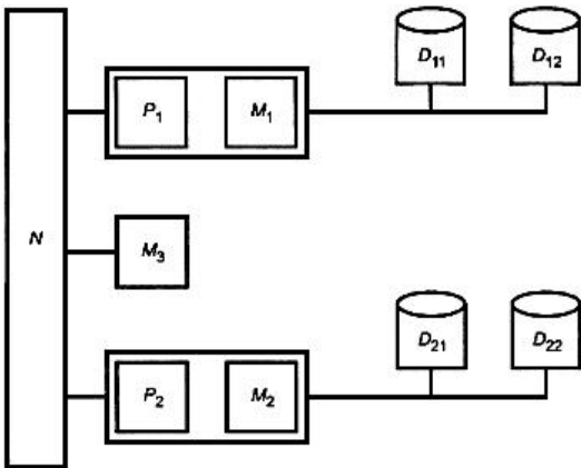
Рисунок А.8 - Структурная схема мультипроцессора
