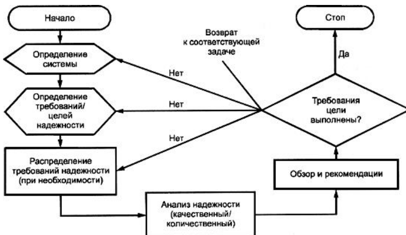
Рисунок 1 - Общая процедура анализа надежности
