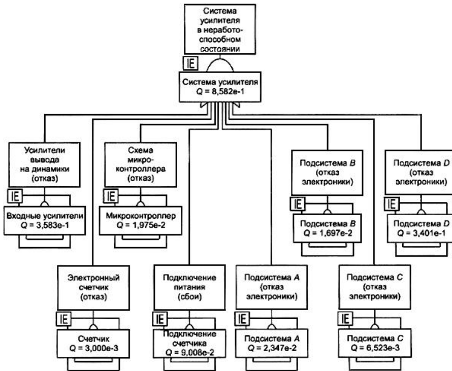
Рисунок А.2 - Дерево неисправностей для аудиоусилителя
