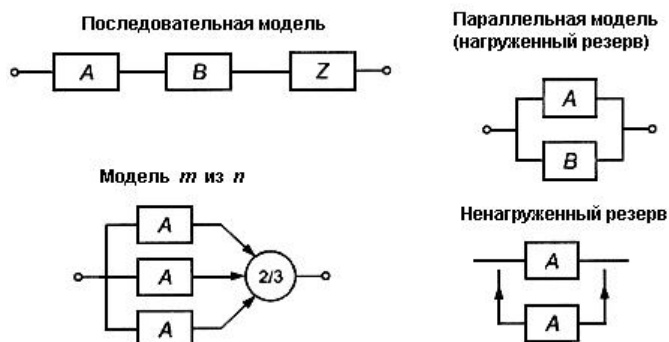
Рисунок А.5 - RBD для независимых блоков
