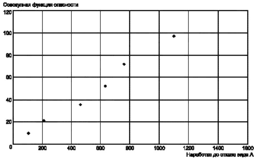
Рисунок А.2 — График совокупной функции опасности
