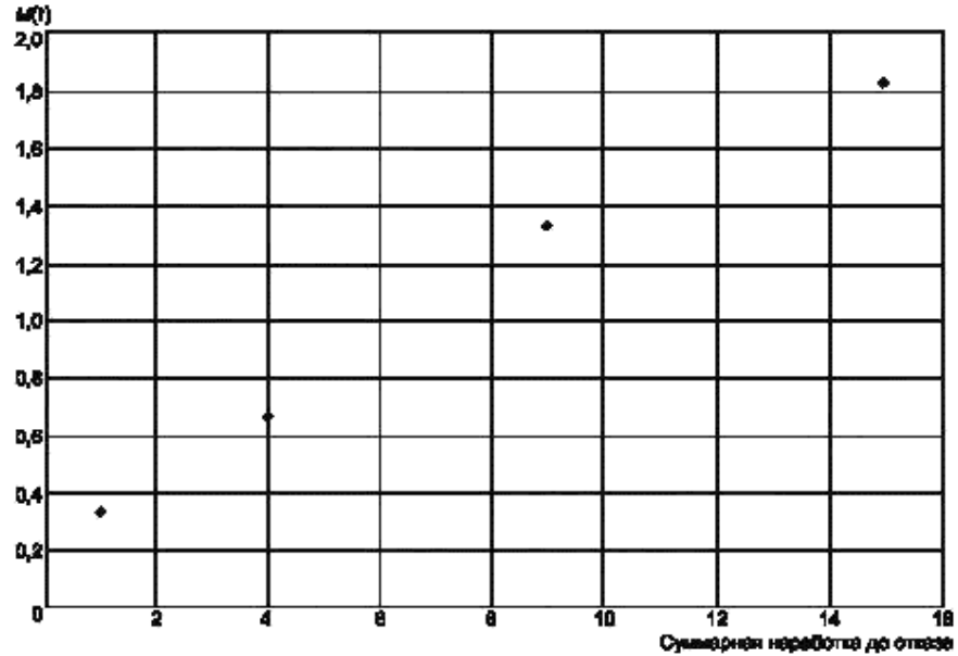
Рисунок А.3 — График M(t) для трех восстанавливаемых объектов
